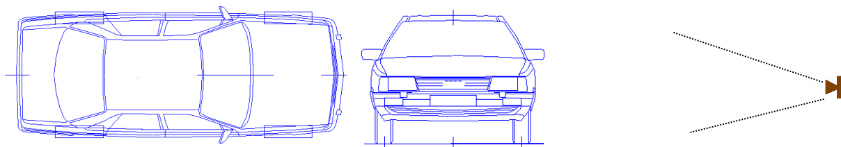
2-сурет. Зақымдалған сол жақтағы алдыңғы есікті фототүсіруді орындау схемасы
