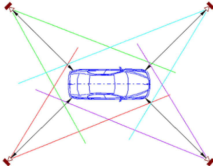
1-сурет. Зақымдалған көлік құралын фототүсіруді орындау схемасы (жалпы түрі)
